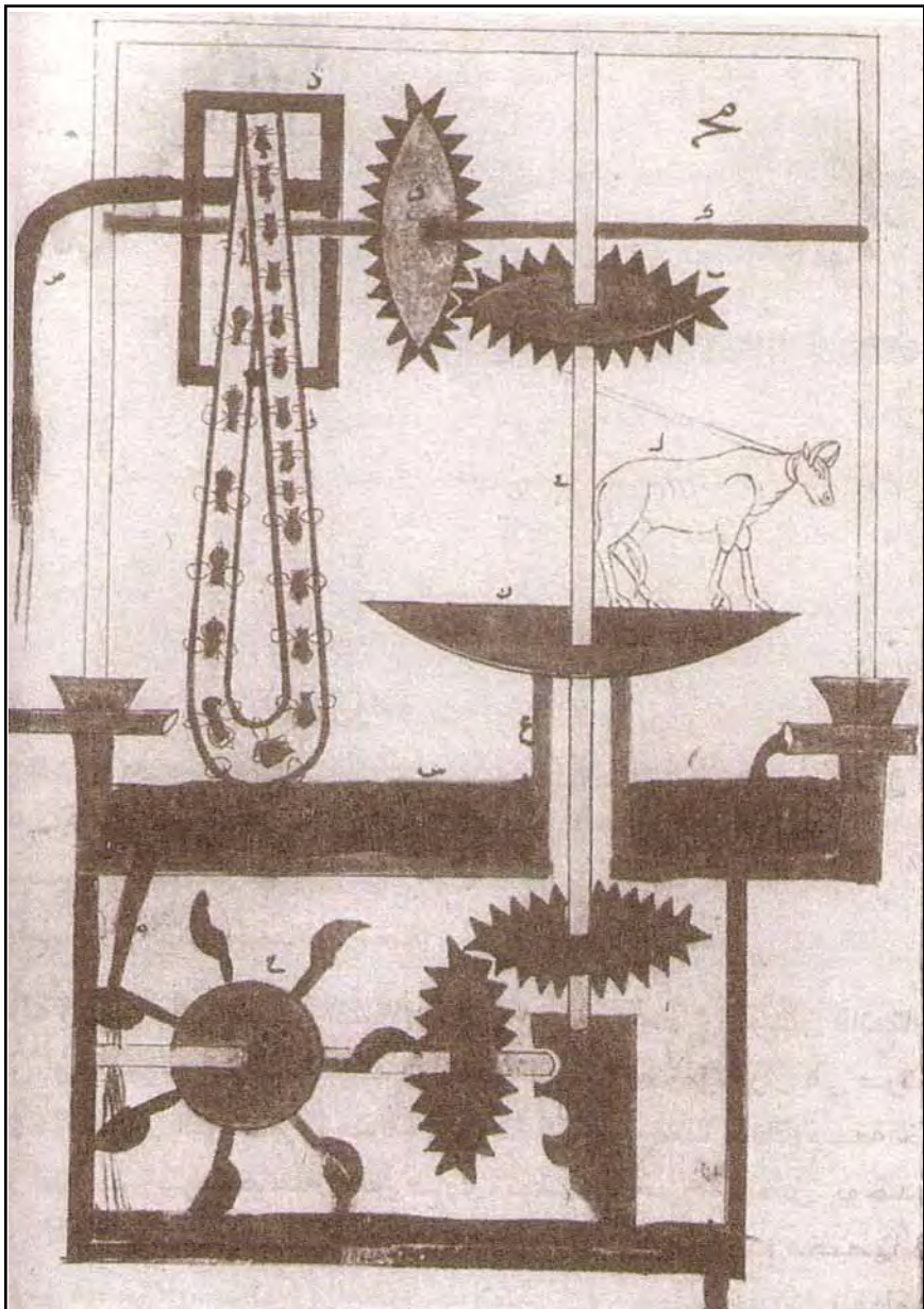
نامبریکی تری بهرز کرده‌وهی ناو له کتیبی (جهزری) یه‌وه بابی پینجه‌م / فه‌صلی س‌یه‌م، نه‌م دانراوه له کتیب‌خانه‌ی (بودنیان) پاریزراوه.
